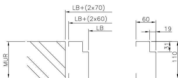
Type D2, cold store, 60/75mm
