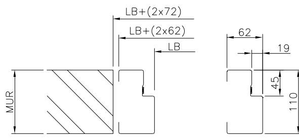
Type D, EI 2 60, cold store, 75 mm
