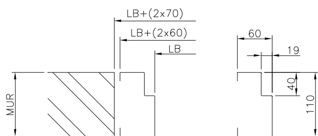
Type D, cold store, 60 mm
