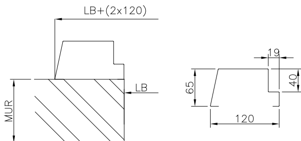
Typ E
