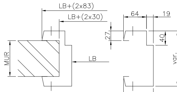
Typ G6
